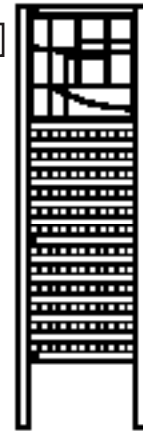
(1) - Panneau de paravent AD - Y70119-019 38,1 x 520,7 x 1676,4 mm
