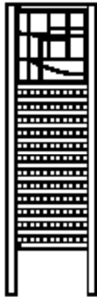
(1) - Panneau de paravent AG - Y70119-018 38,1 x 520,7 x 1676,4 mm
